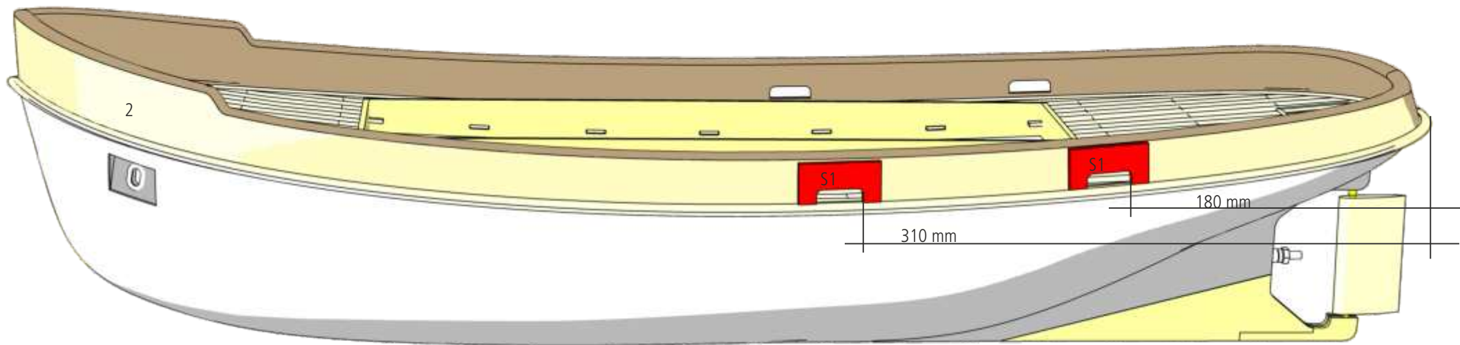
34 Die Schablone S1 auflegen und das Schanzkleid 2 ausschneiden oder fräsen.
