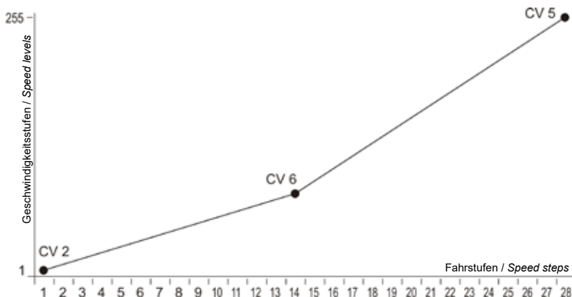
Geschwindigkeitskennlinie nach Vorgabe (CV 2, 5 und 6) Linear characteristic (CV 2, 5 und 6)
